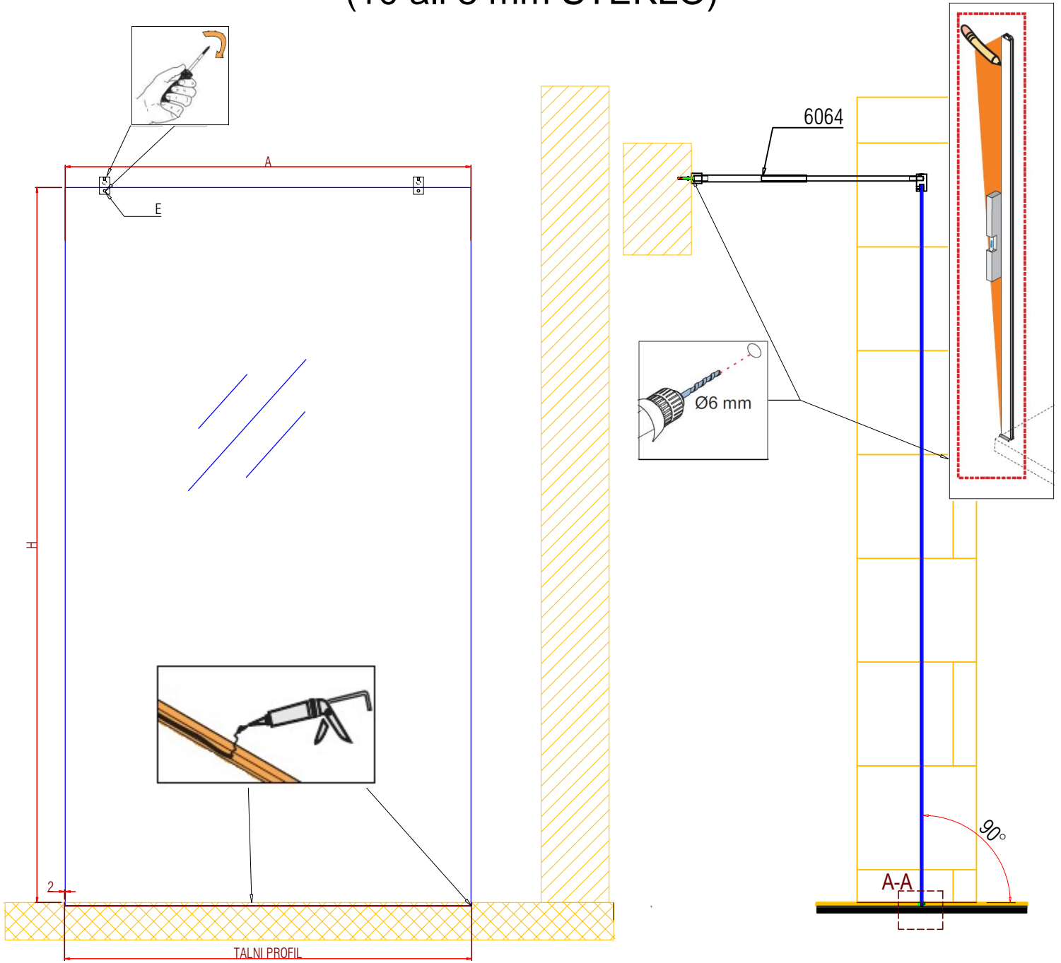
POGLED : A-A
