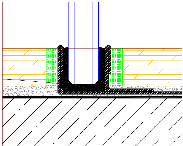
POGLED : A-A
